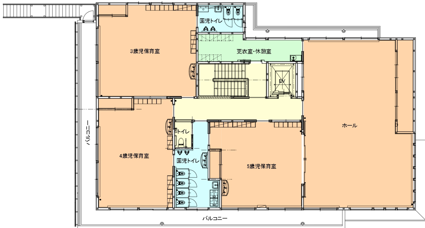
2階平面図
