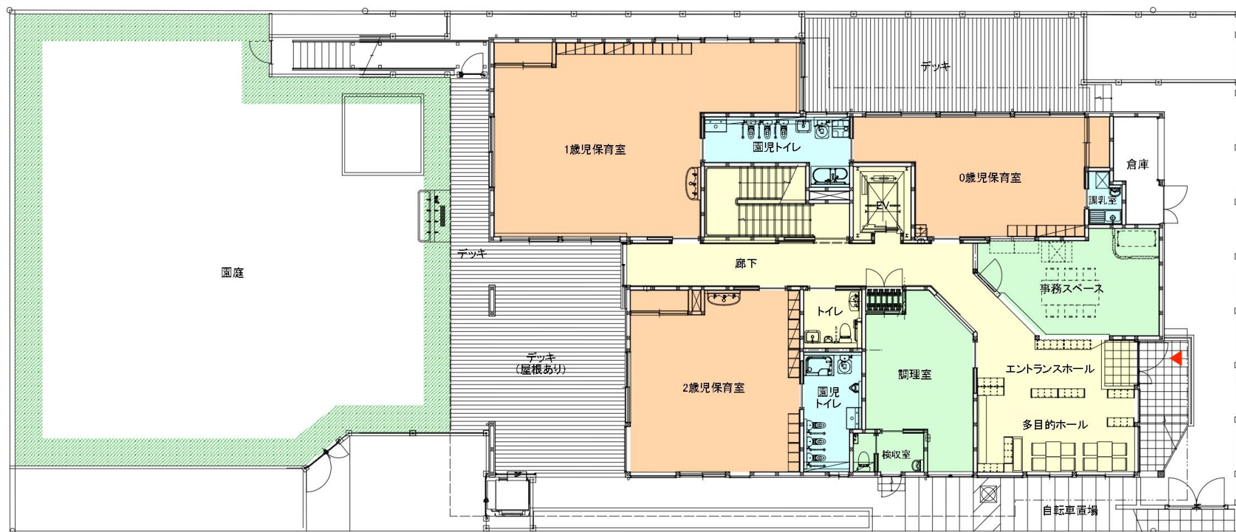
1階平面図
